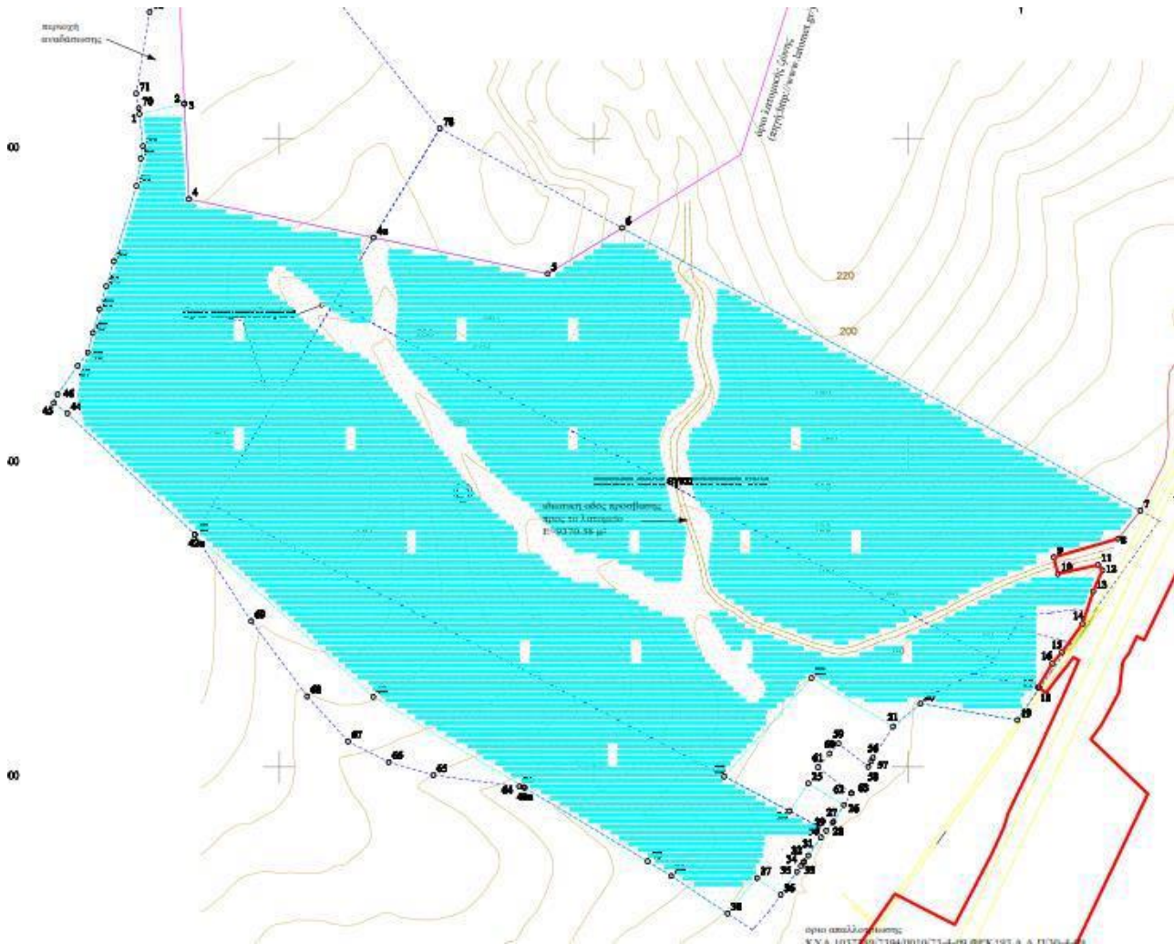
Εικόνα 2-3. Γήπεδο εγκατάστασης του Φ/Β σταθμού, προβλεπόμενη χωροθέτηση των Φ/Β πλαισίων
