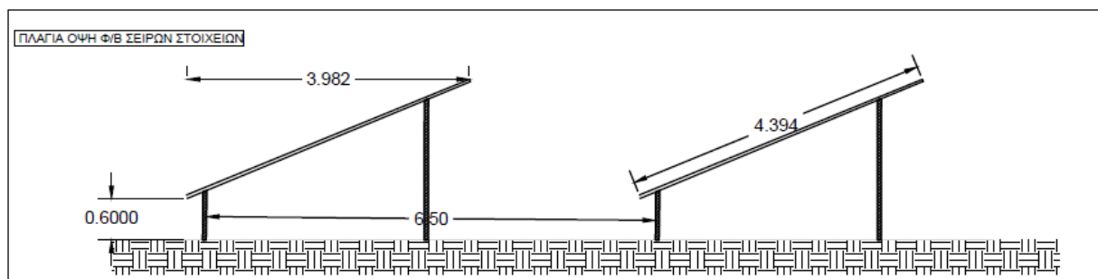
Εικόνα 2-1. Ενδεικτική σχηματική τομή διάταξης Φ/Β πλαισίων
