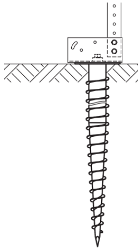
Εικόνα 2-5. Βάσεις στήριξης με πασσαλόμπτυξη
