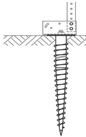
Εικόνα 3-8. Βάσεις στήριξης με πασσαλόμπτυξη
