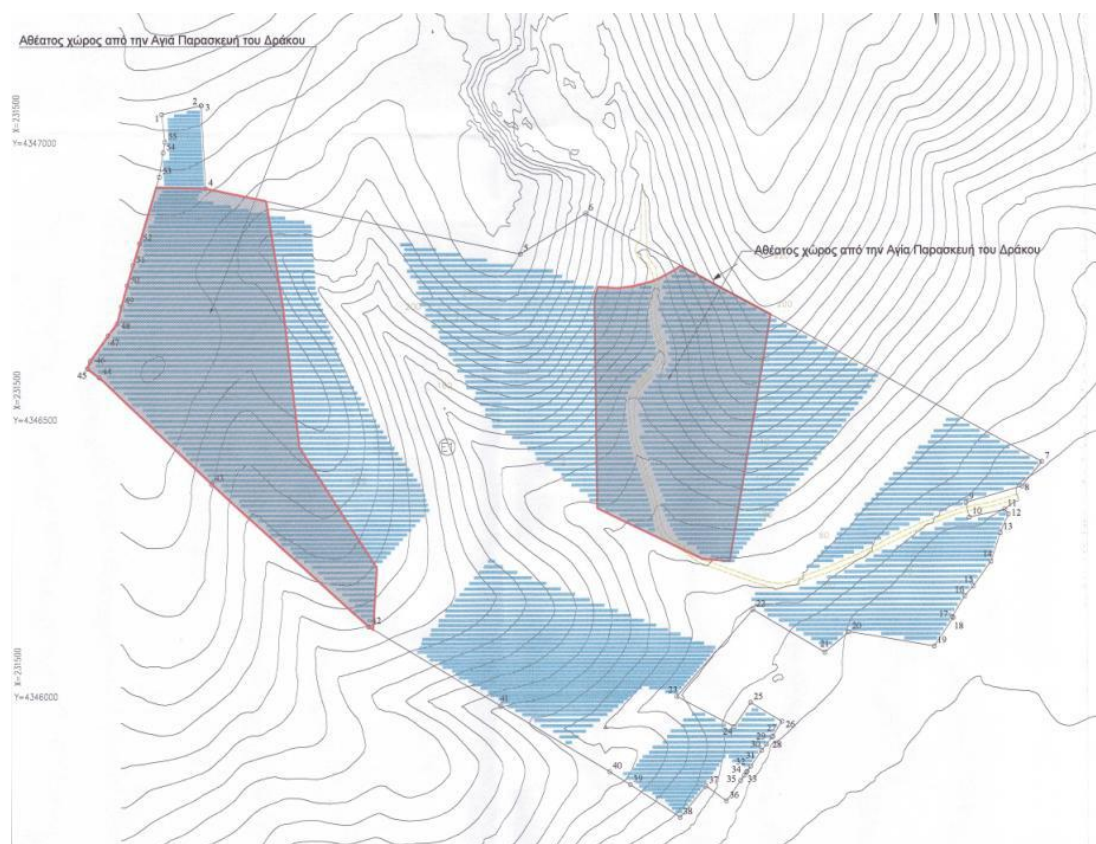
Εικόνα 3-4. Χωροθέτηση Φ/Β πλαισίων
