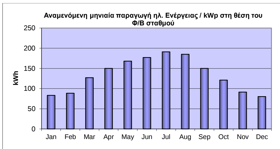
Ετήσια κατανομή παραγωγής ηλεκτρικής ενέργειας
