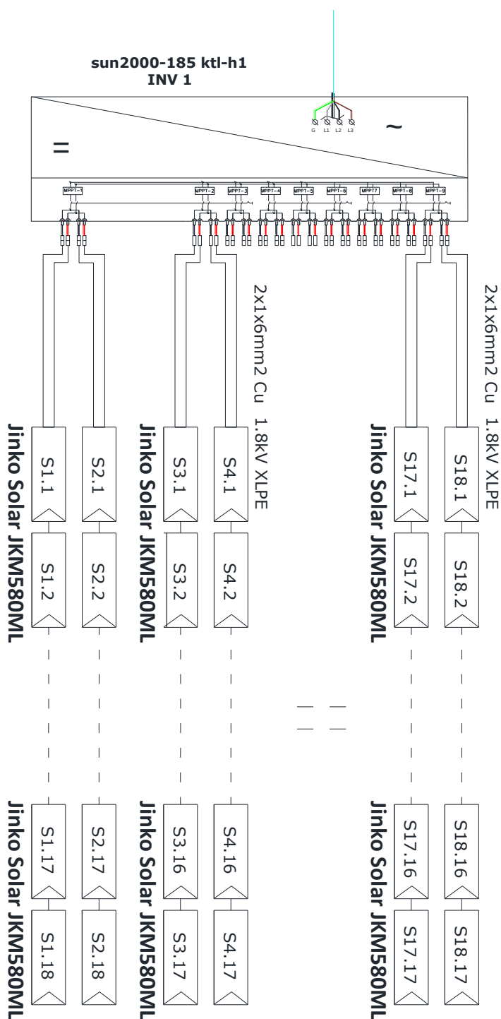
Εικόνα 6.10.: Μονογραμμικό ηλεκτρικό διάγραμμα Χ.Τ. των 8 ομάδων
