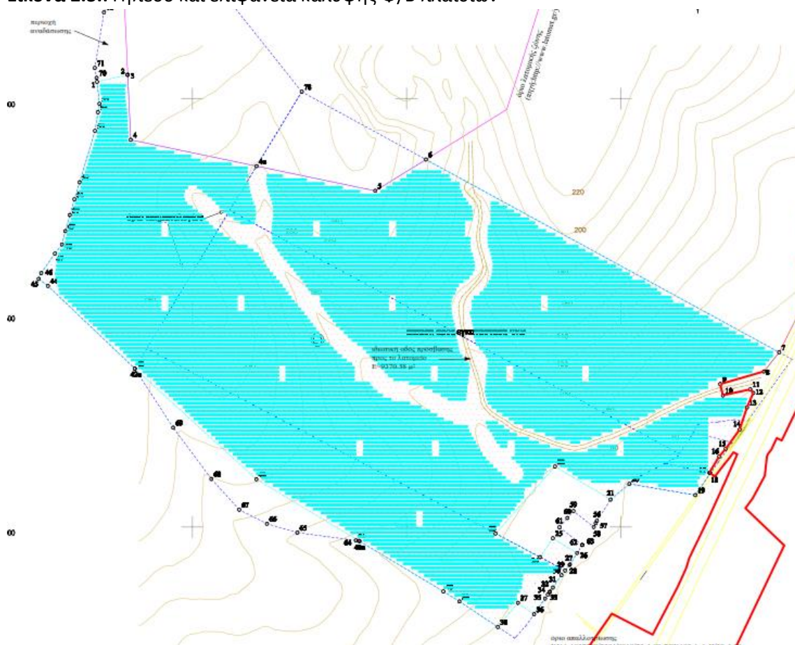
Εικόνα 2.3.: Γήπεδο και επιφάνεια κάλυψης Φ/Β πλαισίων
